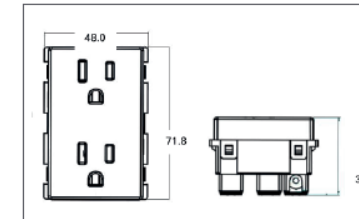
Figura 4. Tomacorriente sencillo
