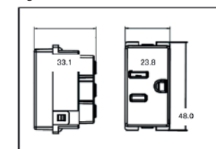
Figura 4. Tomacorriente sencillo
