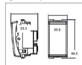
Figura 3. Interruptores
